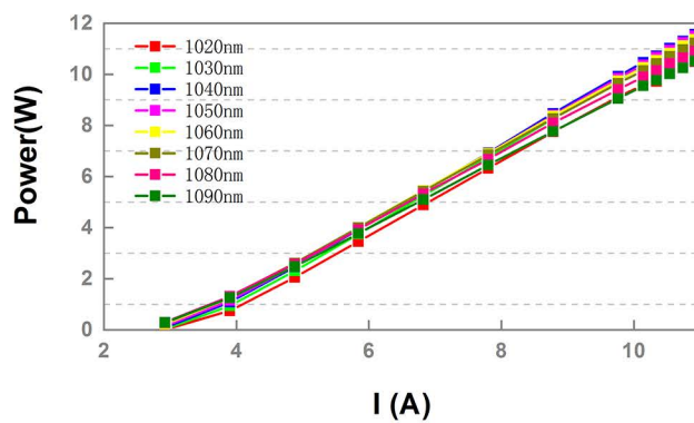
输出功率
