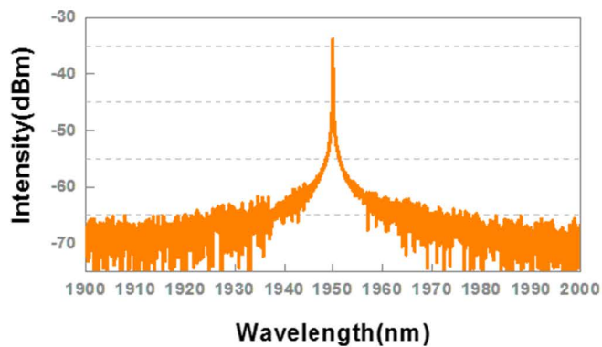
典型输出光谱
